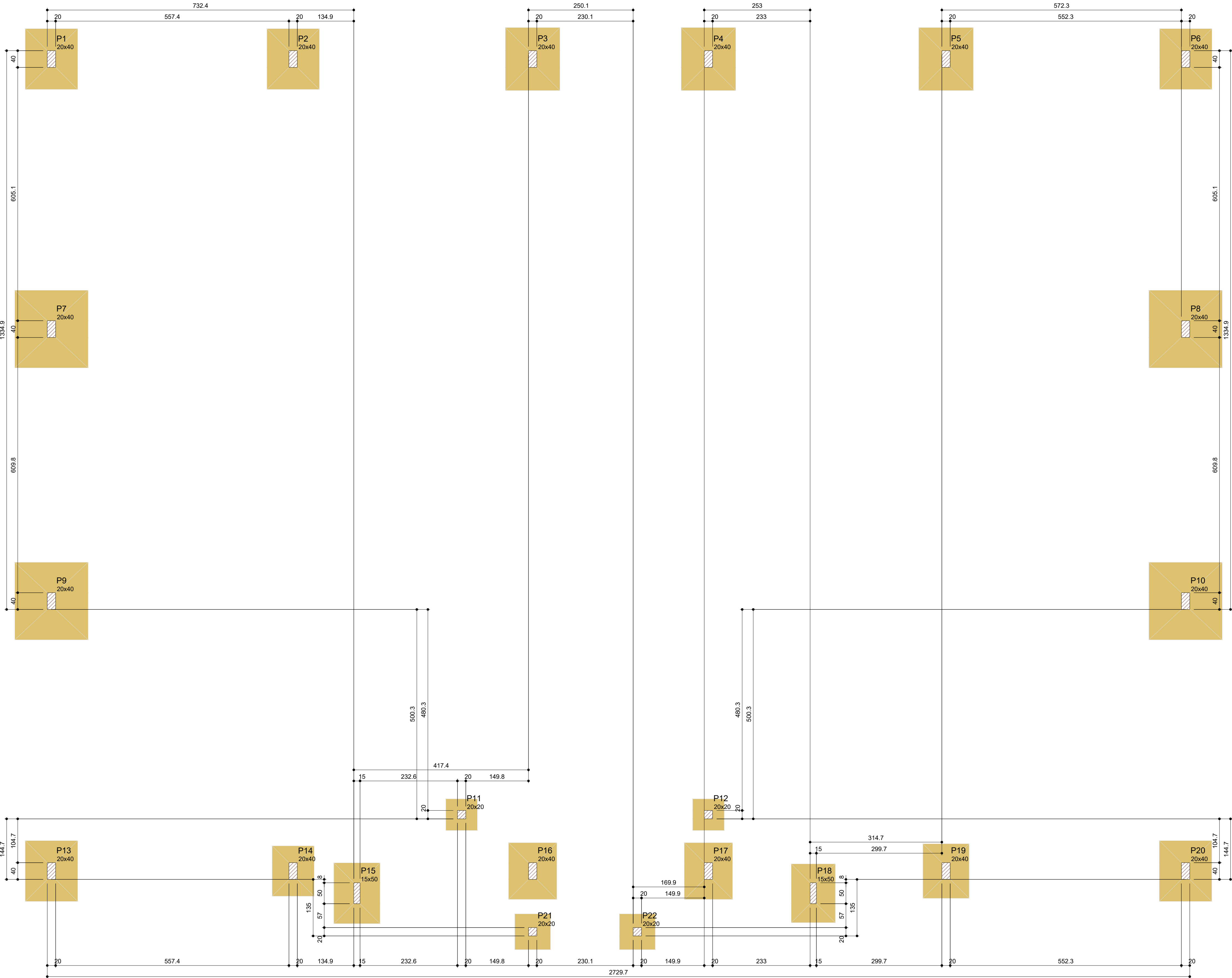
Forma do pavimento Fundação (Nível 0) escala 1:50
