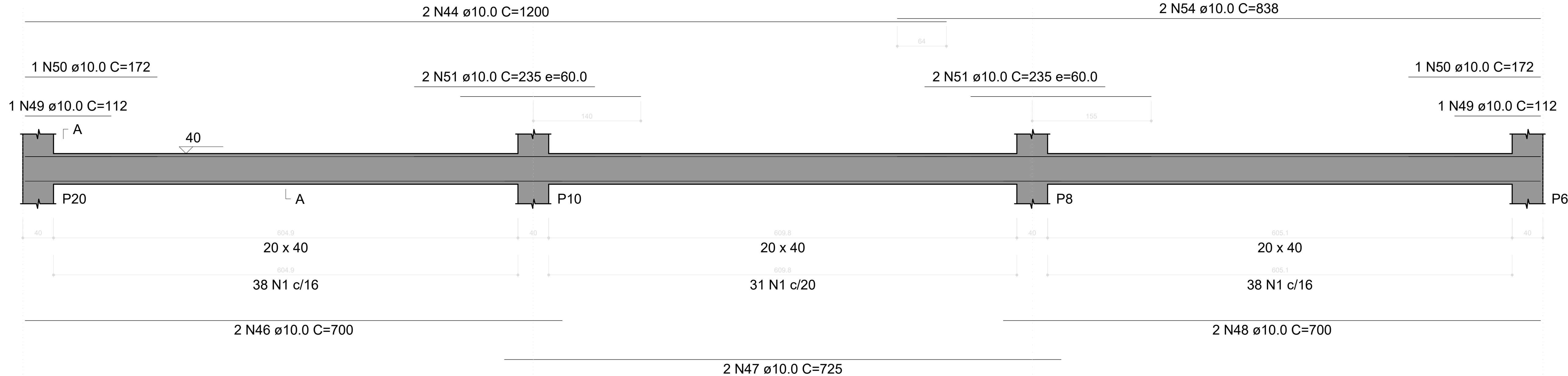
V14 ESC 1:30
