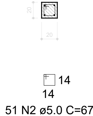
SEÇÃO A-A ESC 1:25
