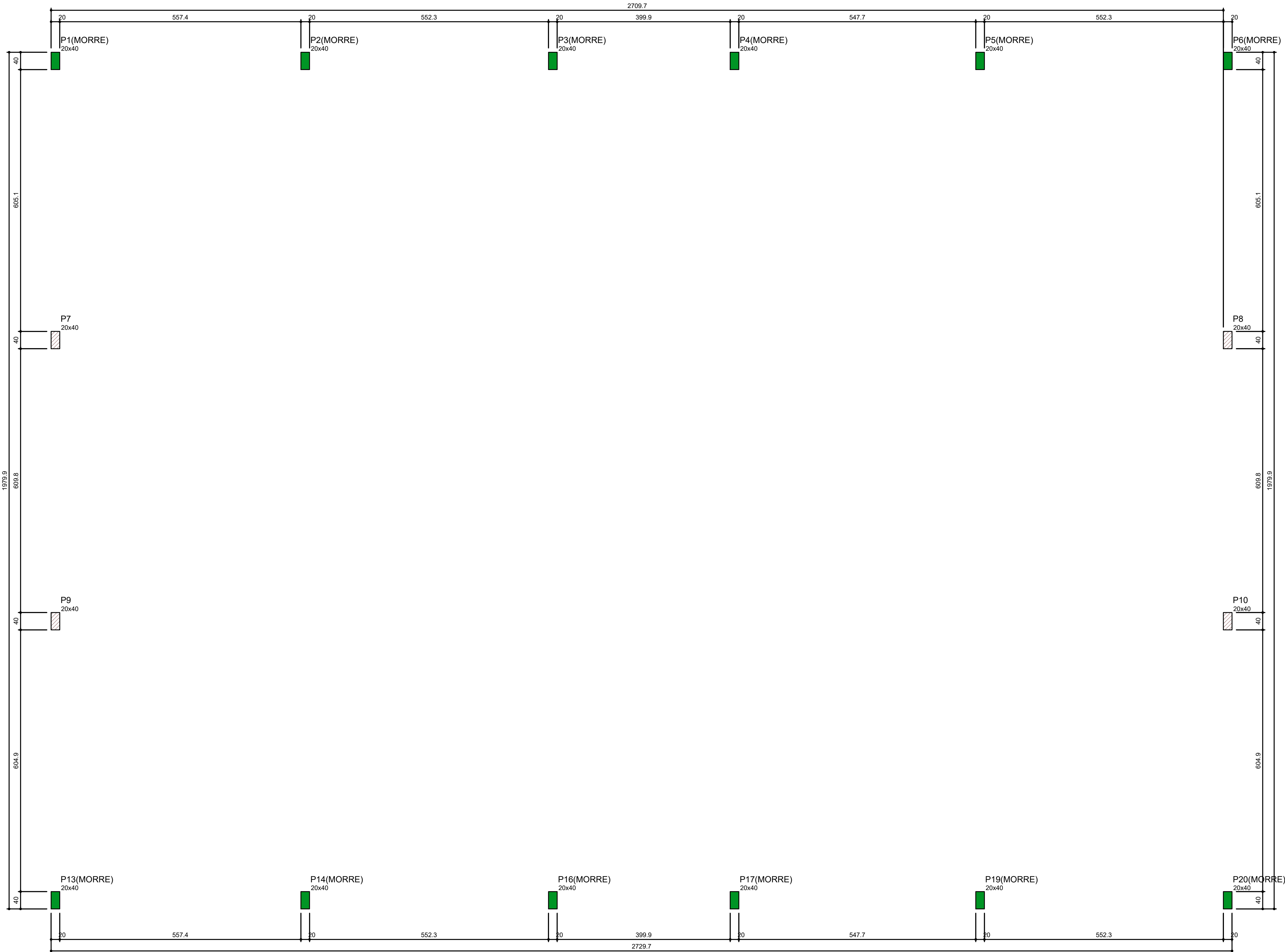
Forma do pavimento Térreo (Nível 330) escala 1:50
