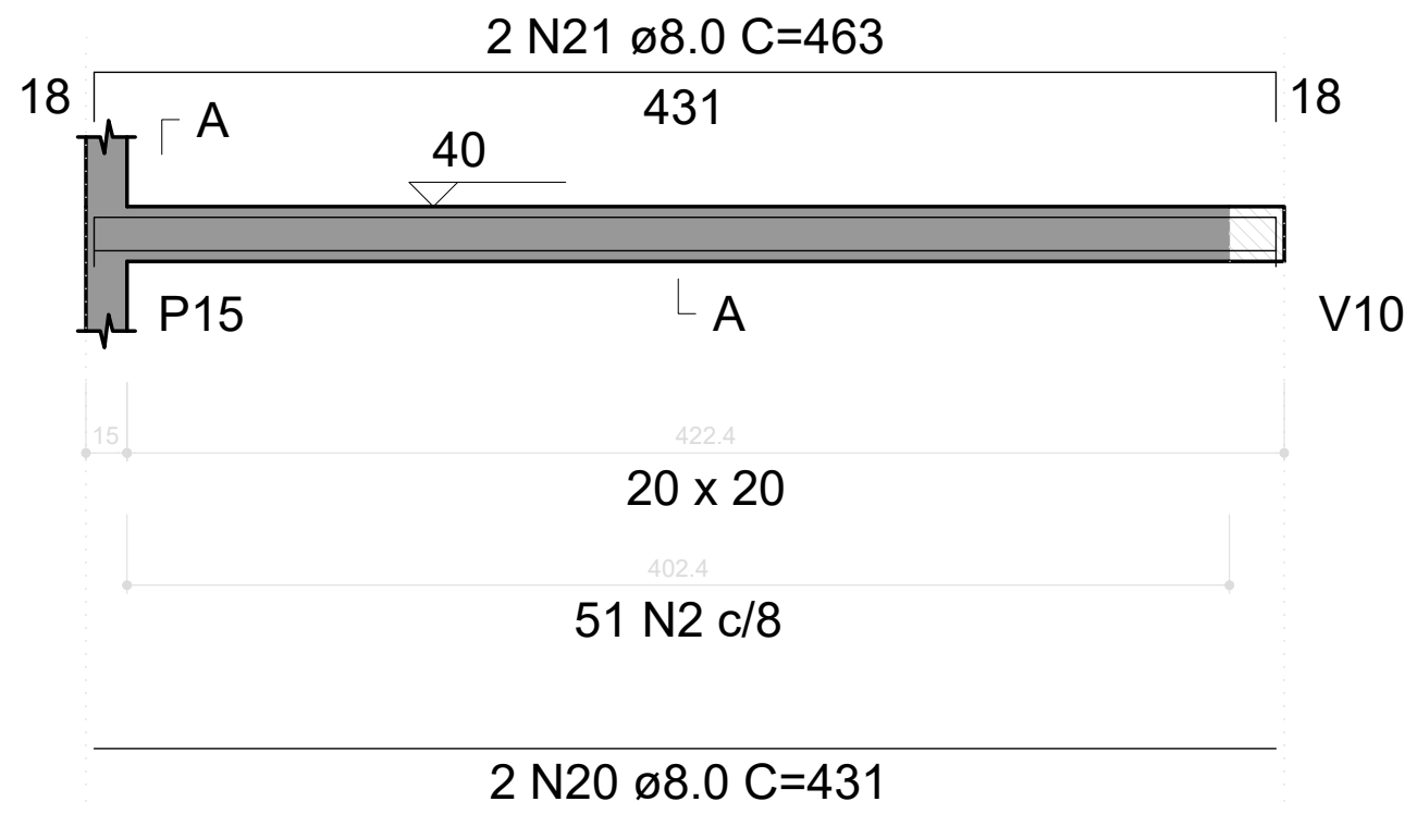
V4 ESC 1:30
