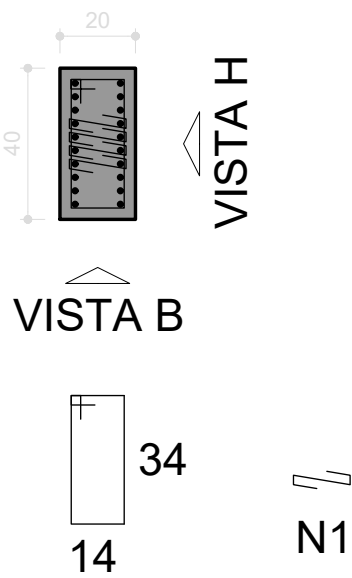
SEÇÃO ESC 1:20
