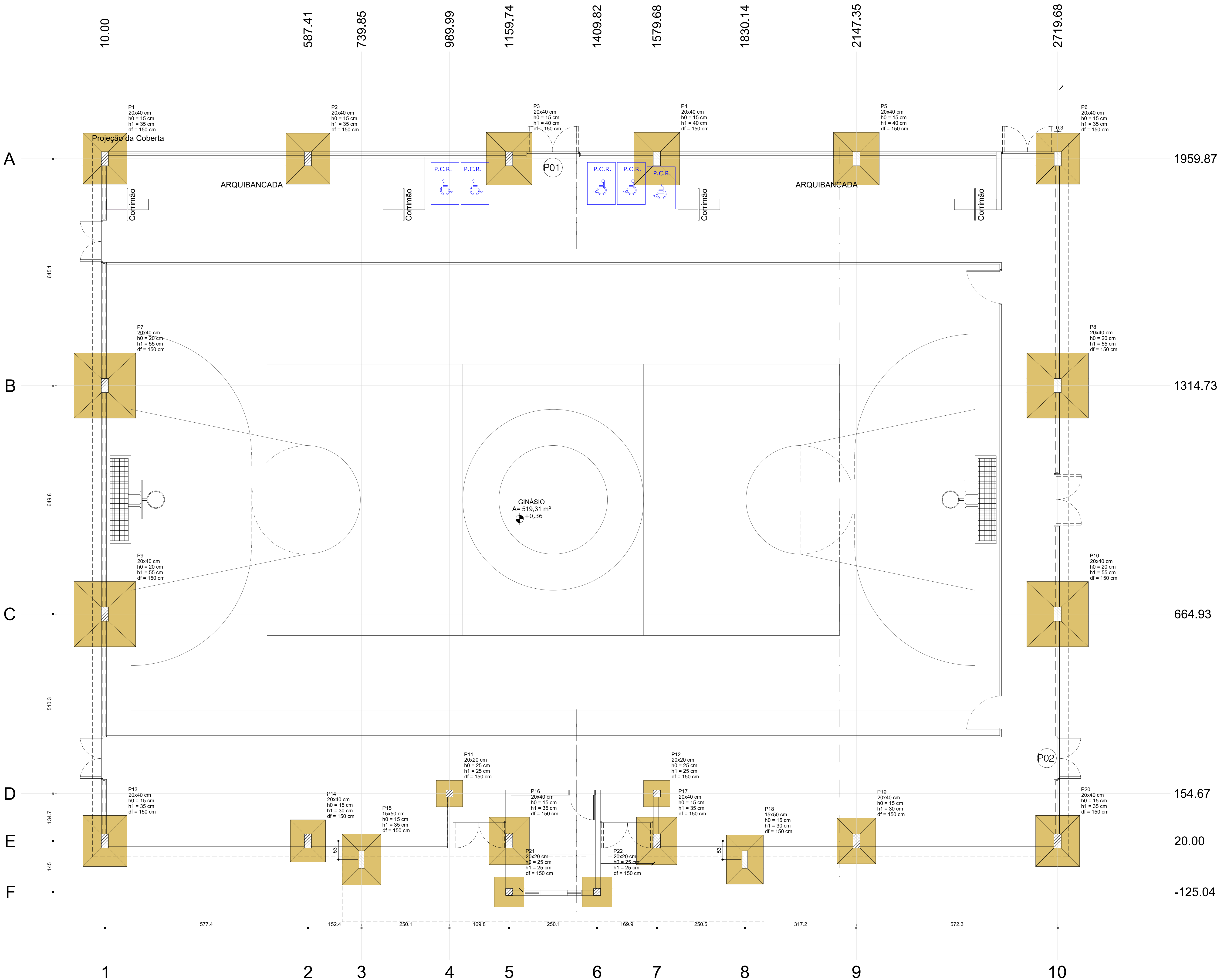
Planta de locação escala 1:50
