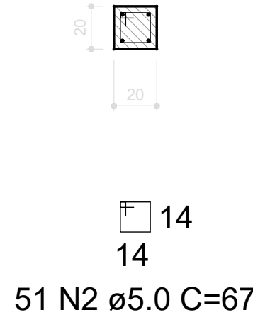
SEÇÃO A-A ESC 1:25
