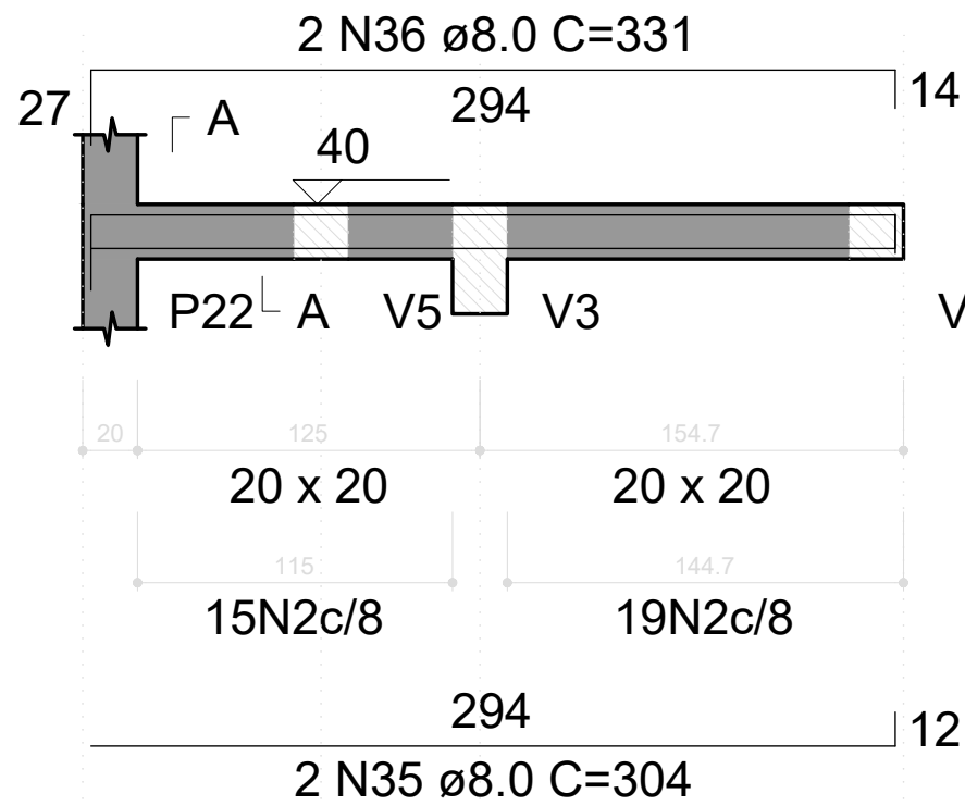
SEÇÃO A-A ESC 1:25
